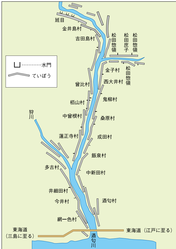
酒匂川の流れてにそってきずかれたていぼう (「とみず子ども風土記」より)
